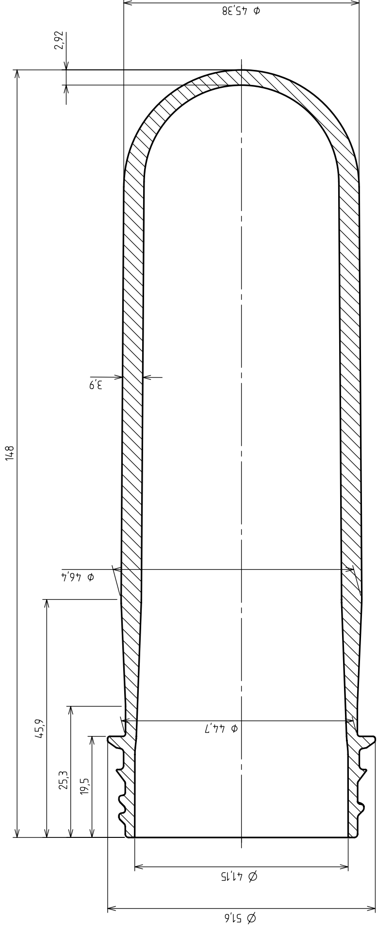
SECTION A-A SCALE 2:1
