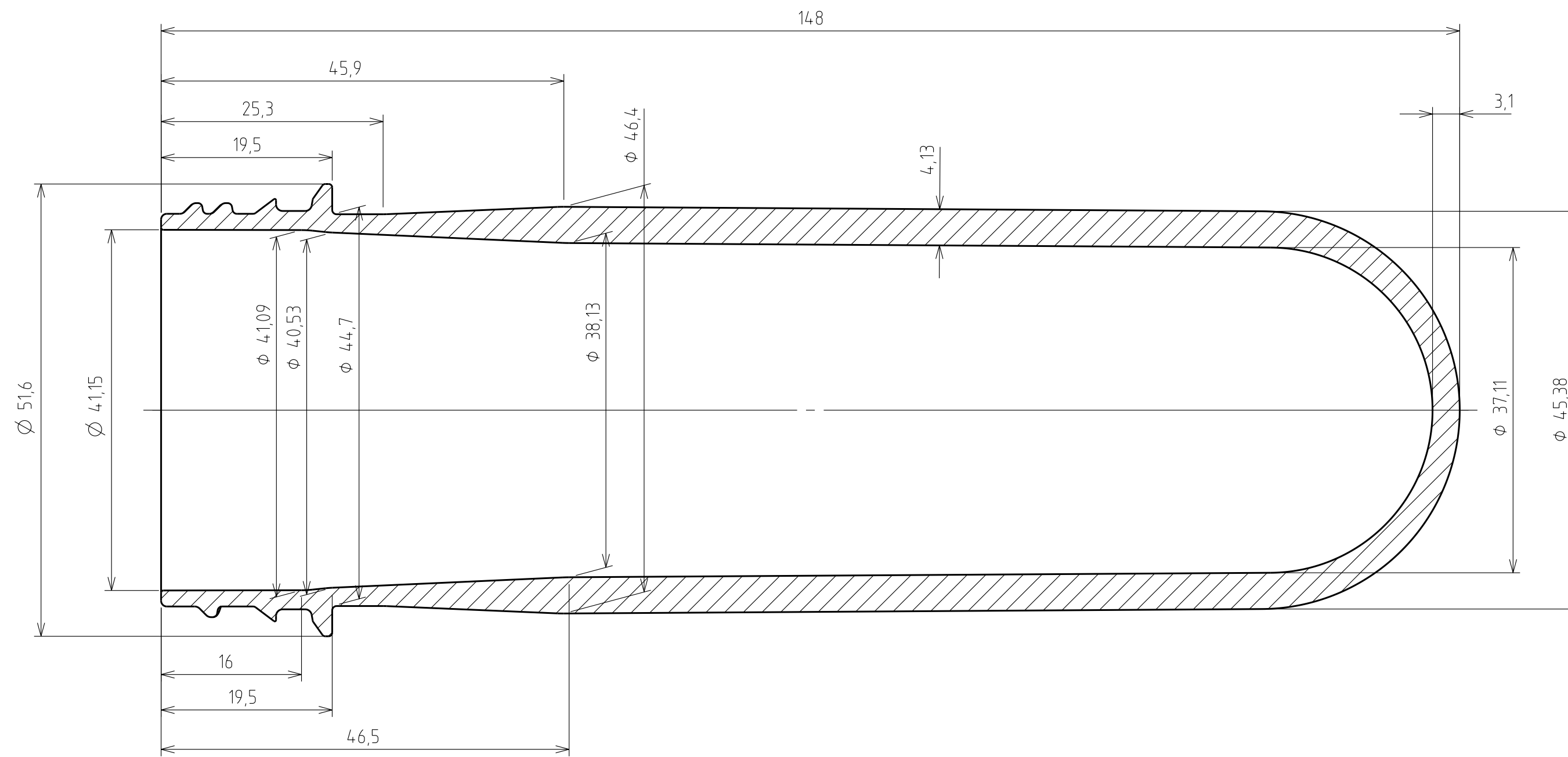
SECTION A-A SCALE 2:1
