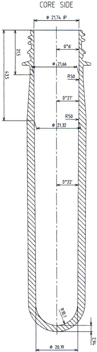
SECTION A-A SCALE 2:1
