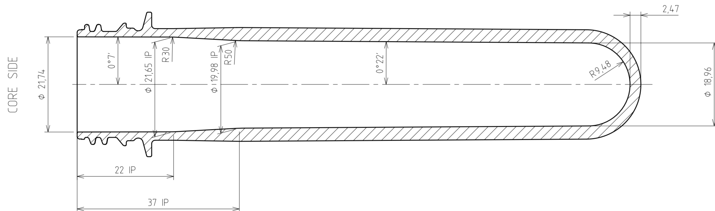
SECTION A-A SCALE 2:1
